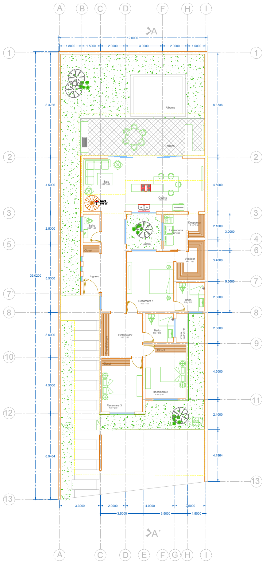
Planta arquitectonica Esc: 1:100
